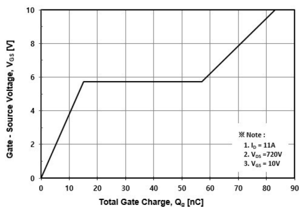
Fig. 6 V_{GS} - Q_G
