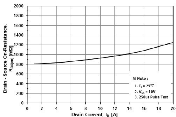
Fig. 3 R_{DS(ON)} - I_D
