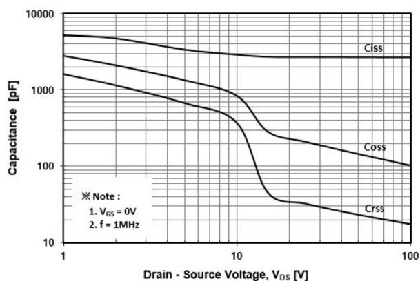
Fig. 5 Capacitance - V_{DS}
