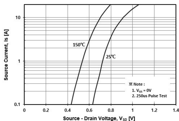
Fig. 4 I_S - V_{SD}
