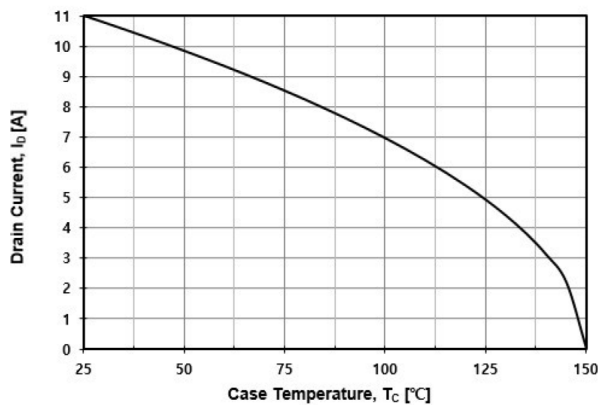
Fig. 9 I_D - T_C
